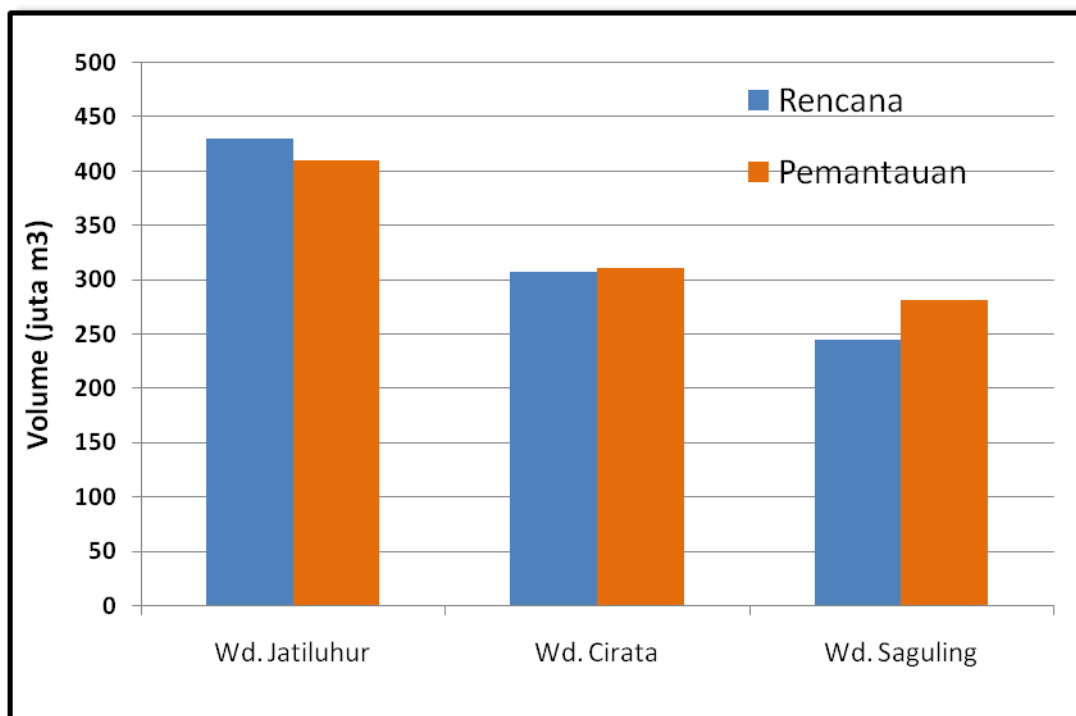
Gambar 3. Perbandingan Volume Rencana dan Pemantauan 3 Waduk Utama di Jawa Barat (Status 15 s/d 28 Februari 2019)
