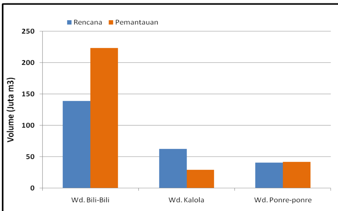
Gambar 6. Perbandingan Volume Rencana dan Pemantauan 3 Waduk Utama di Sulawesi Selatan (Status 15 s/d 28 Februari 2019)
