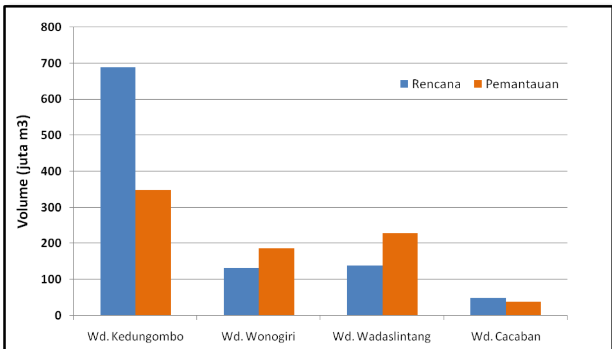
Gambar 4. Perbandingan Volume Rencana dan Pemantauan 4 Waduk Utama di Jawa Tengah (Status 15 s/d 28 Februari 2019)
