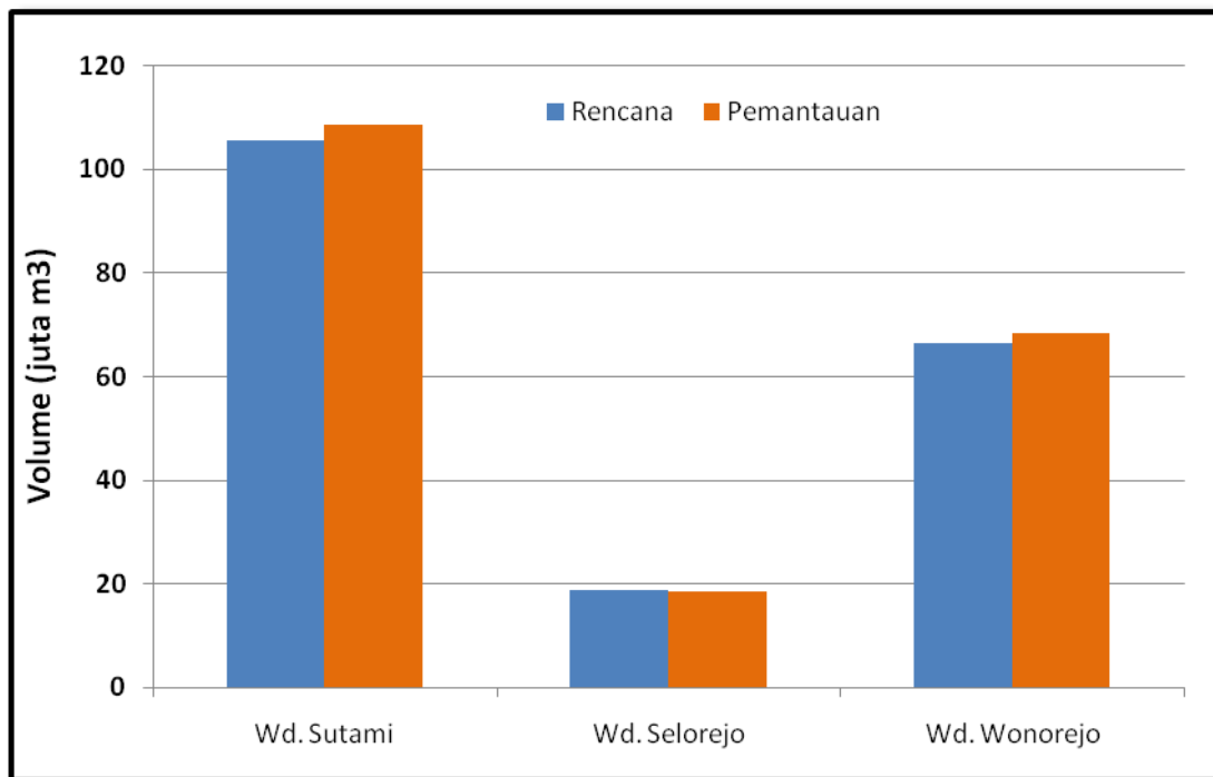
Gambar 5. Perbandingan Volume Rencana dan Pemantauan 3 Waduk Utama di Jawa Timur (Status 15 s/d 28 Februari 2019)
