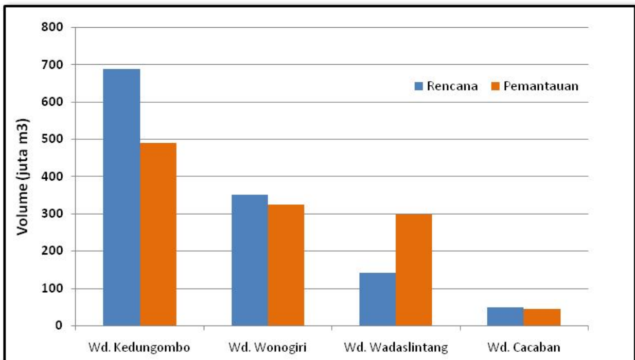
Gambar 4. Perbandingan Volume Rencana dan Pemantauan 4 Waduk Utama di Jawa Tengah (Status 15 s/d 30 April 2019)
