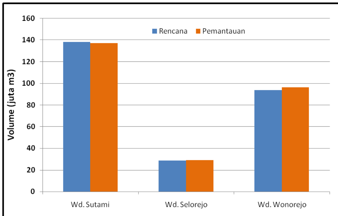
Gambar 5. Perbandingan Volume Rencana dan Pemantauan 3 Waduk Utama di Jawa Timur (Status 15 s/d 30 April 2019)
