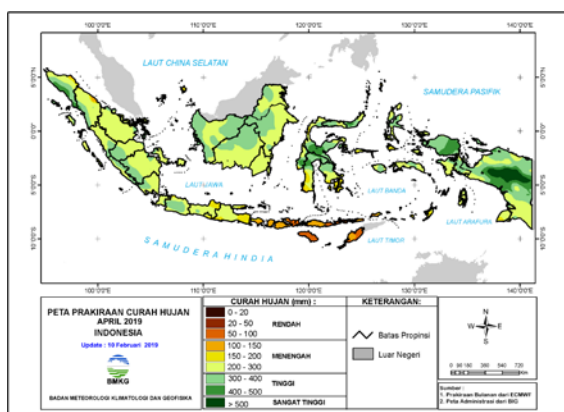
1a. Prakiraan Curah Hujan April 2019
