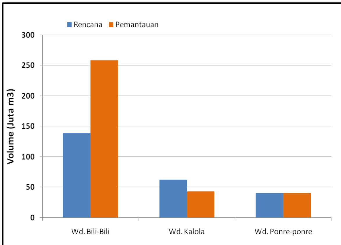
Gambar 6. Perbandingan Volume Rencana dan Pemantauan 3 Waduk Utama di Sulawesi Selatan (Status 15 s/d 30 April 2019)
