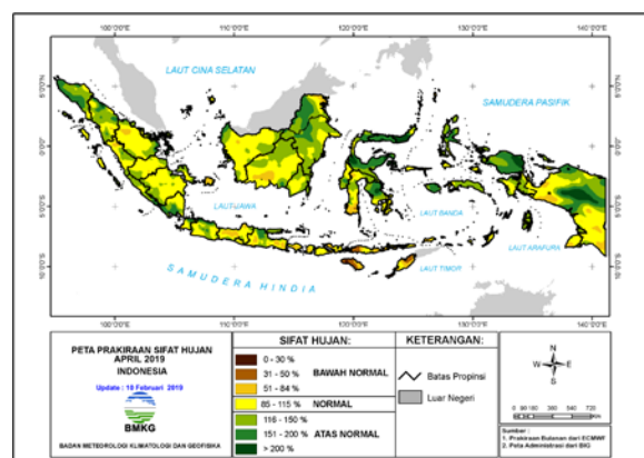
1b. Prakiraan Sifat Hujan April 2019
