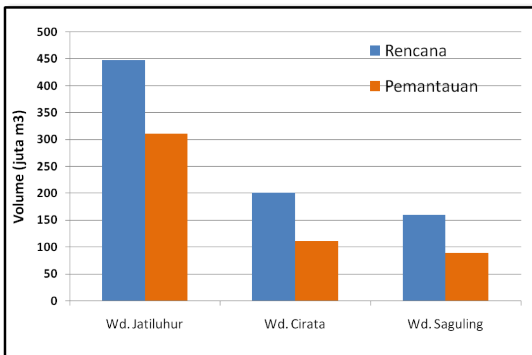
Gambar 3. Perbandingan Volume Rencana dan Pemantauan 3 Waduk Utama di Jawa Barat (Status 15 s/d 30 September 2019)
