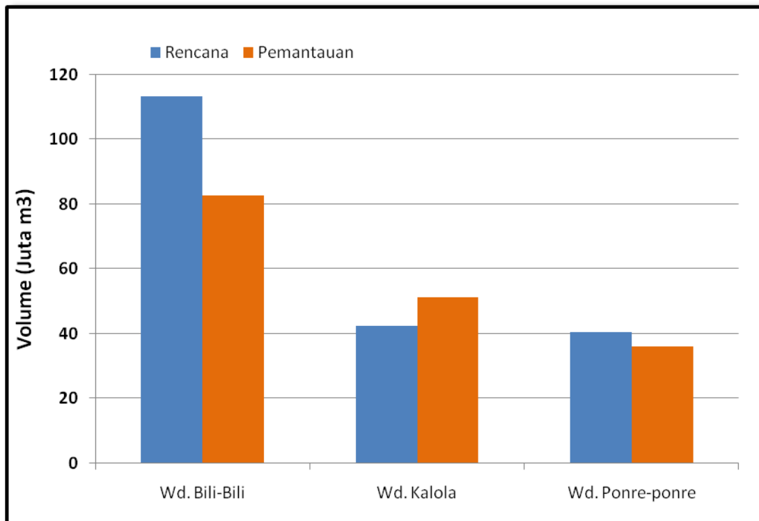
Gambar 6. Perbandingan Volume Rencana dan Pemantauan 3 Waduk Utama di Sulawesi Selatan (Status 15 s/d 30 September 2019)
