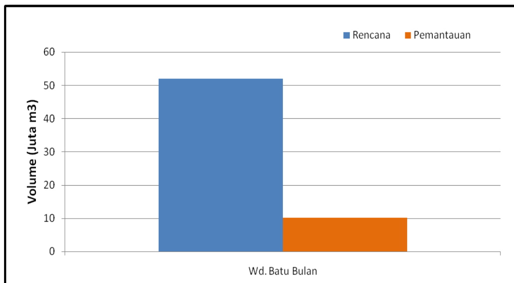
Gambar 7. Perbandingan Volume Rencana dan Pemantauan Waduk Batu bulan di NTB (Status 15 s/d 30 September 2019)
