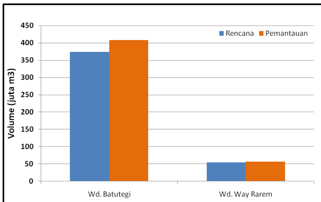
Gambar 8. Perbandingan Volume Rencana dan Pemantauan 2 Waduk utama di Lampung (Status 15 s/d 30 September 2019)
