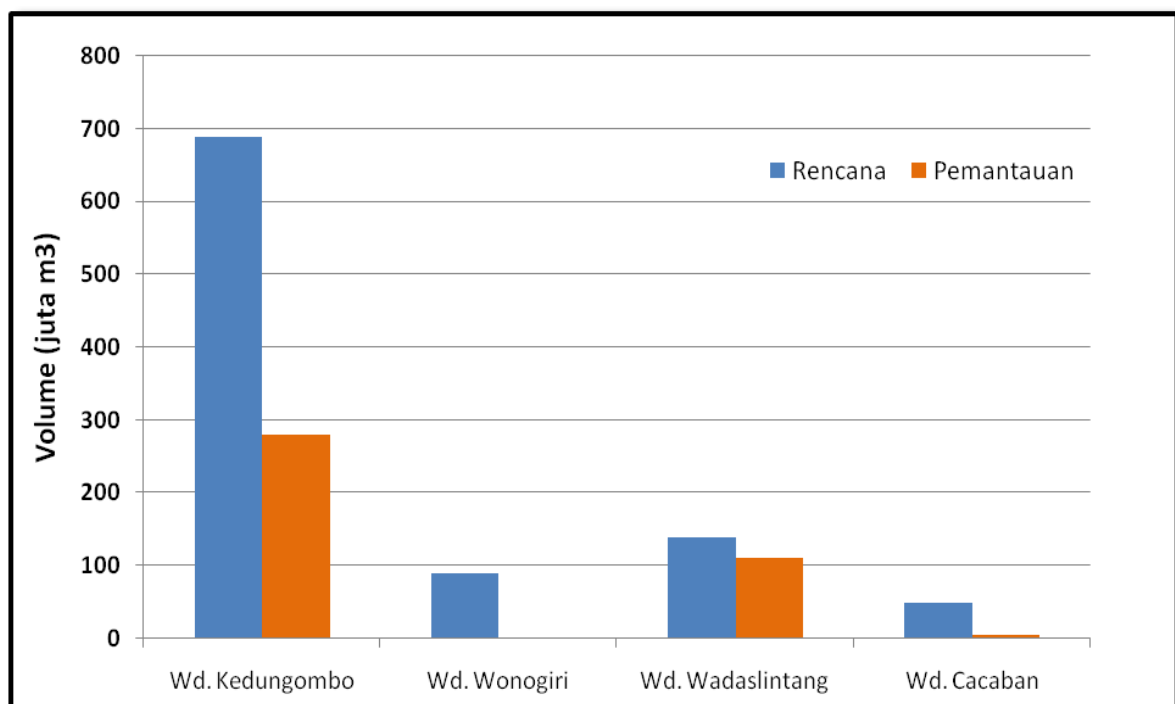
Gambar 4. Perbandingan Volume Rencana dan Pemantauan 4 Waduk Utama di Jawa Tengah (Status 15 s/d 30 September 2019)
